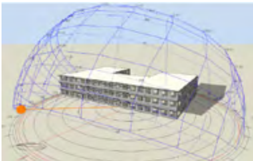
Export depuis le logiciel DesignBuilder. © Inddigo
