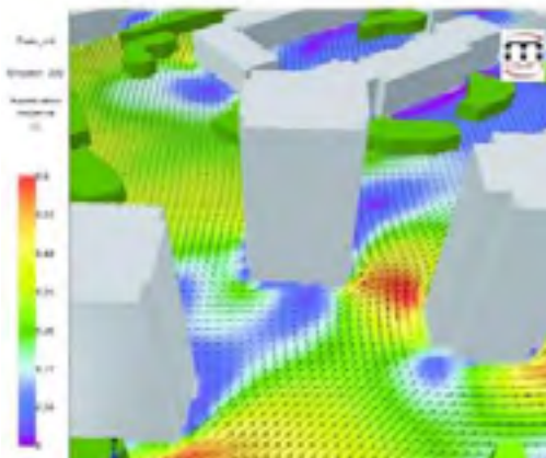
Représentation graphique des fréquences et vitesses de vent dans l'espace public. © Meteodyn
