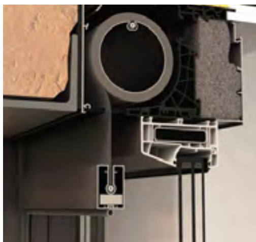
Détail de store zippé résistant au vent © RENSON
