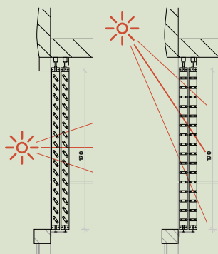
Détail balcon type 3 - Éch. 1/50°
