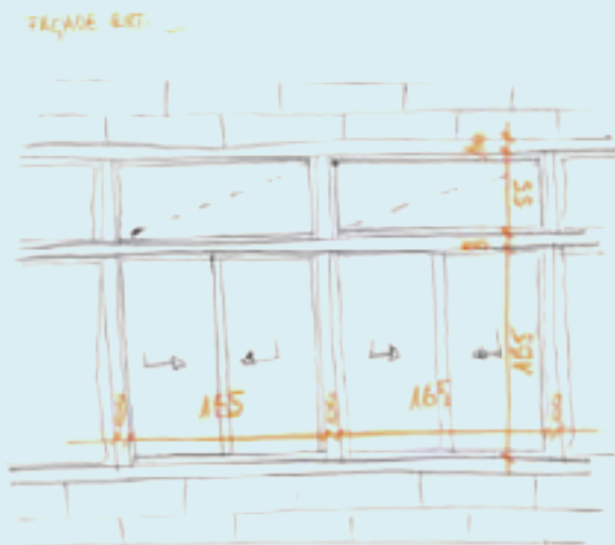
Coupe et façade existantes
