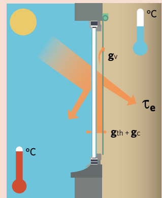
Cas d'une protection solaire intérieure déployée
