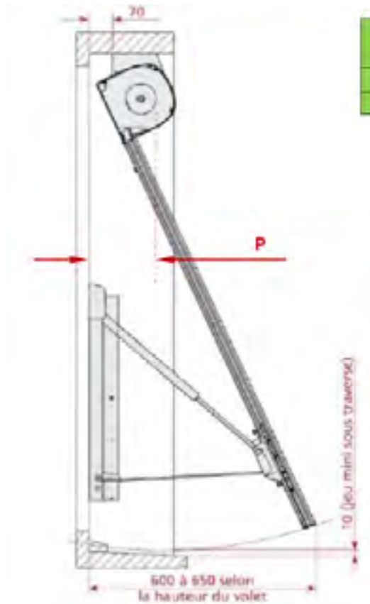
Schéma en coupe de montage © Franciaflex
