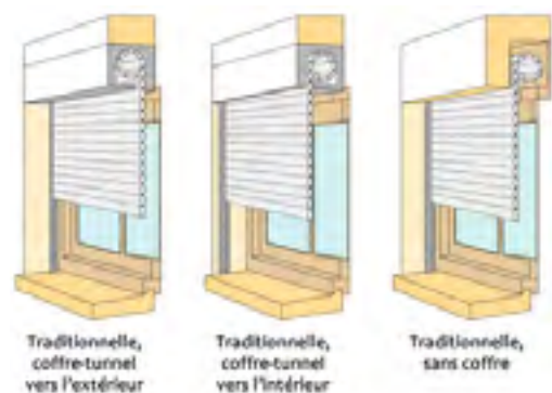
Différents types de pose de volets roulants
