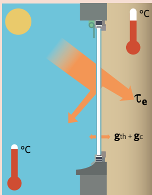
Cas d'une protection solaire relevée
