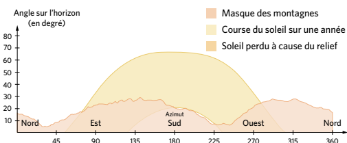
Représentation graphique des masques lointains sur course du soleil orthographique
