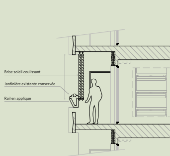
Détail balcon type 3 - Éch. 1/50°
