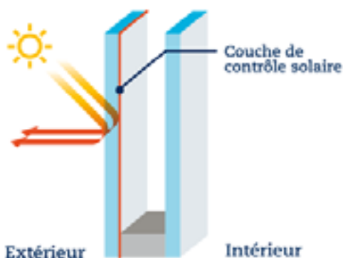
Les vitrages à contrôle solaire. © Fécamp Services
