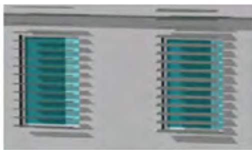
Modélisations sous Pleiades et analyse des ombres portées et insolation des façades.
