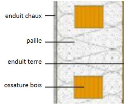
Parois étudiées en ACV statique et dynamique
