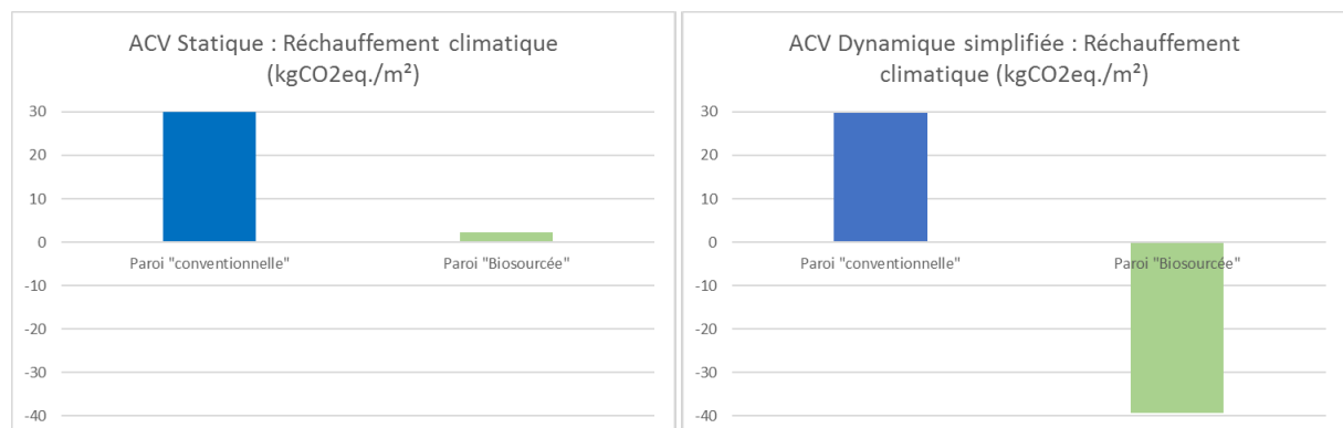
Impact sur le réchauffement climatique par m 2 de paroi (base Inies® décembre 2020) – ACV statique vs dynamique simplifiée
