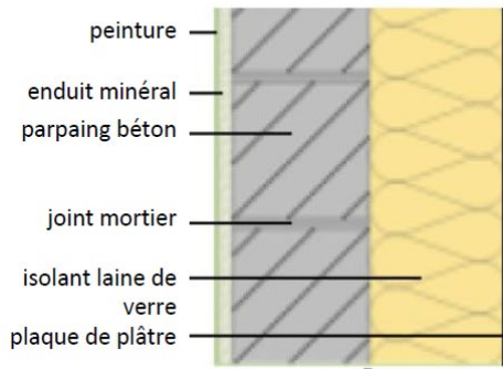
Parois étudiées en ACV statique et dynamique
