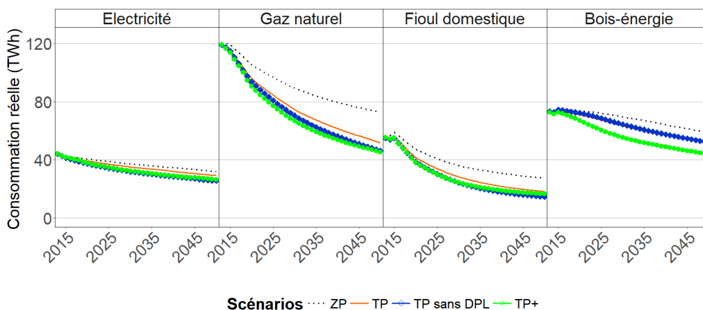
Figure 34: Consommation totale d'énergie réelle
