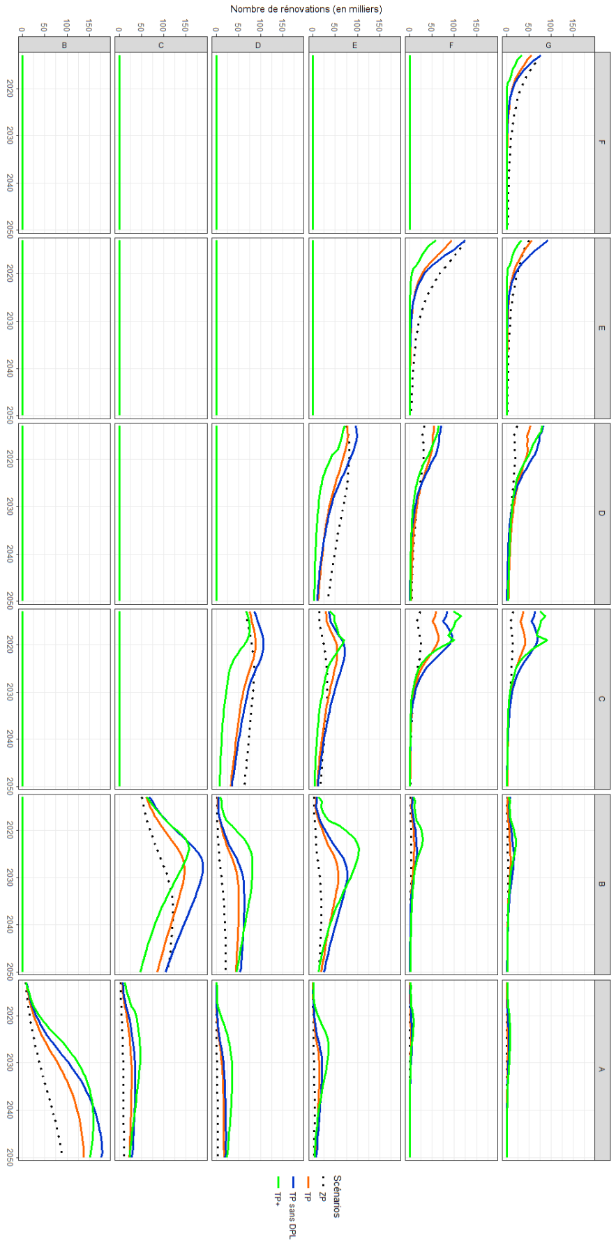
Figure 42: Transitions d'étiquette
