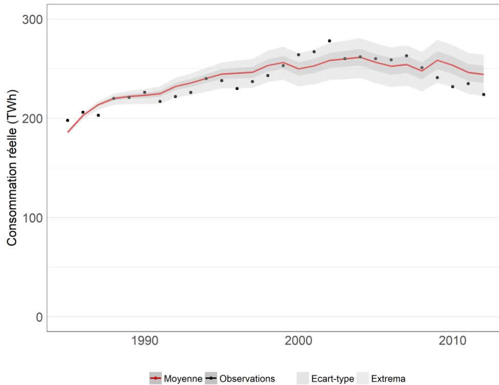
Figure 32: Evolution des consommations simulées et observées
