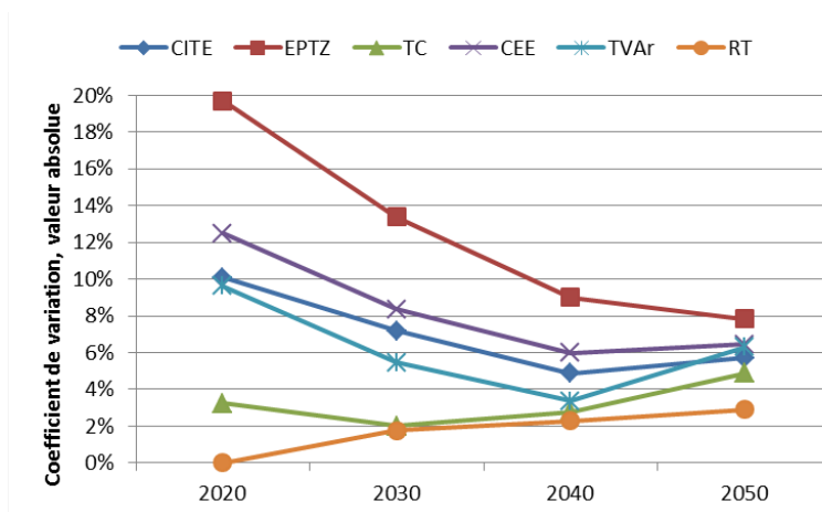
Figure 53: Coefficients de variation en énergie conventionnelle
