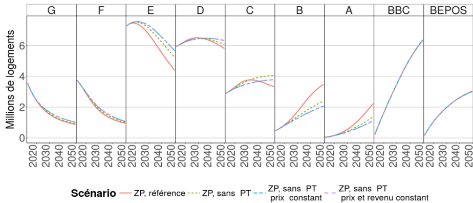
Figure 17: Evolution de la performance énergétique du parc
