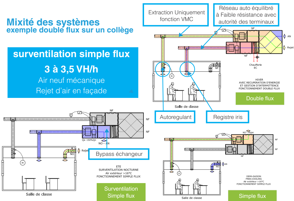
Figure 25 : exemple scolaire système mixte
