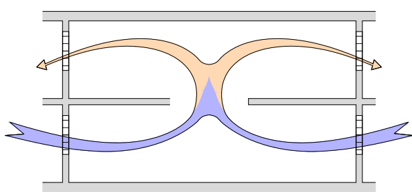
Figure 7 : tirage thermique
