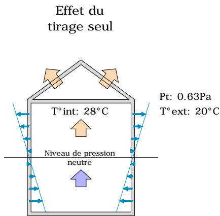
Figure 20 : effet du tirage thermique seul
