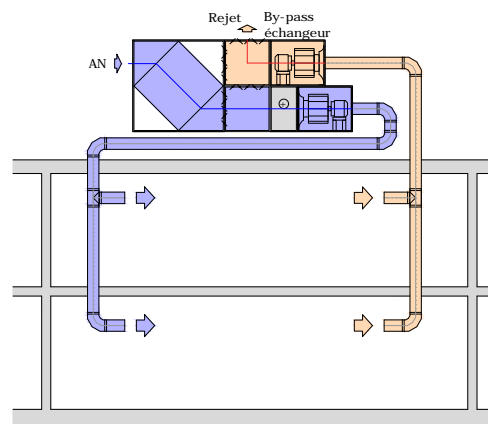
Figure 4 : traitement d'air avec by-pass de l'échangeur
