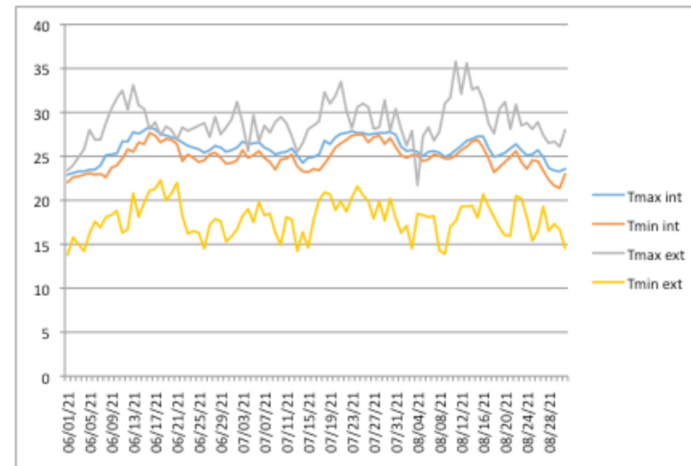
Etage Nord
